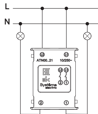
Двухполюсный ВЫКЛЮЧАТЕЛЬ
